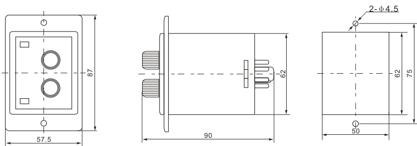
ATDV-N外形图
