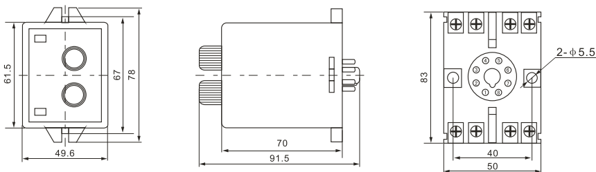
ATDV-N外形图
